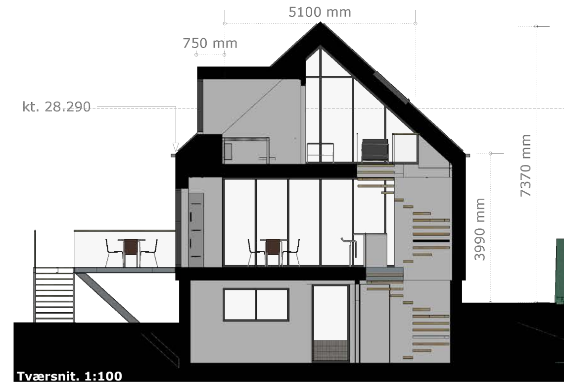
Tværsnit. 1:100
