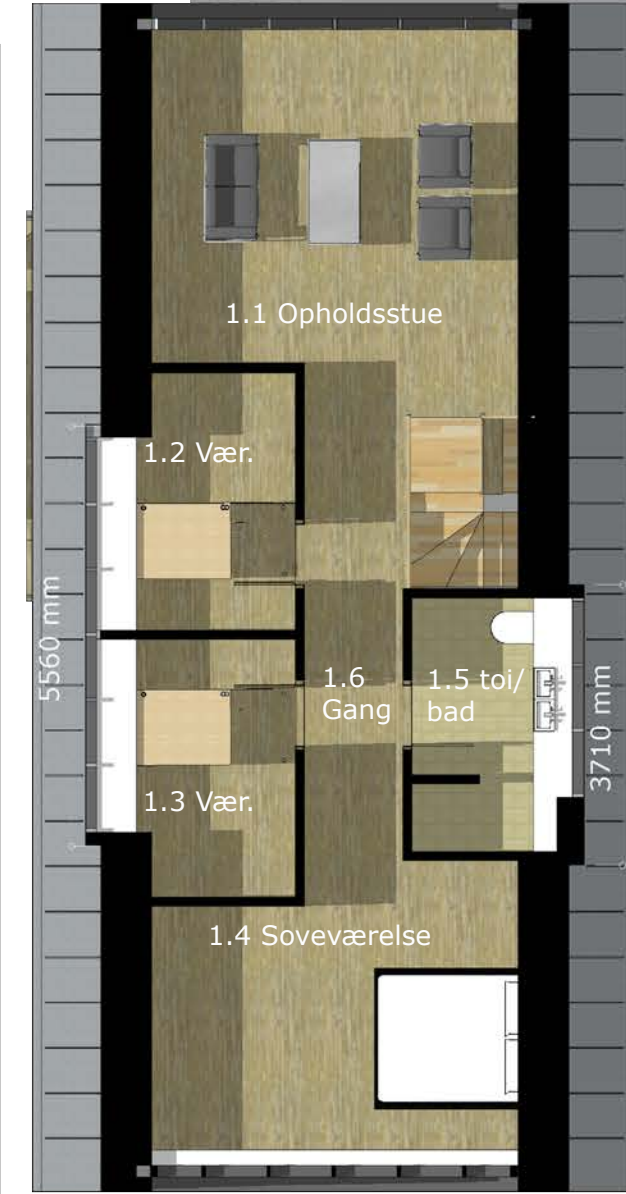
1. Salsplan. 1:100
