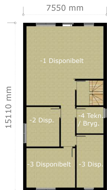
Kælderlan. 1:200
